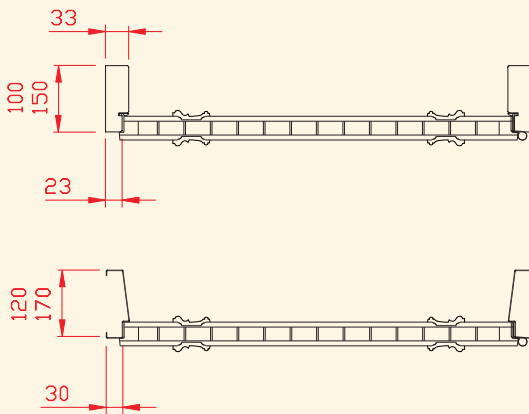
SECCIONES HORIZONTALES DE PUERTAS - CORTE B
